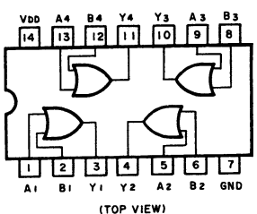
Fig. 8.1.4 OR Gate C-MOS IC \mu PD4071BC
