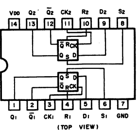
Fig. 8.1.5 D-Type Flip-Flop C-MOS IC \mu PD4013BC
