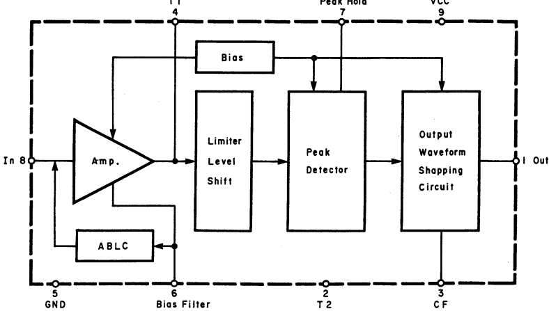
Fig. 8.1.10 Pre-amp. IC \mu PC1474HA
