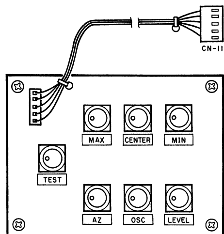
Fig. 5.2 Test Unit
